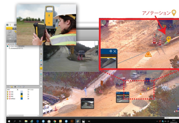
Trimble RealWorks 上でのアノテーションの表示
