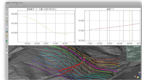
メッシュと縦断 / 横断面を同時に表示
