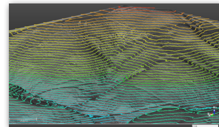
任意の設定で素早くコンタ作成
